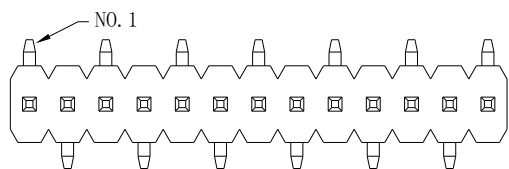
Single row - M1 Type
